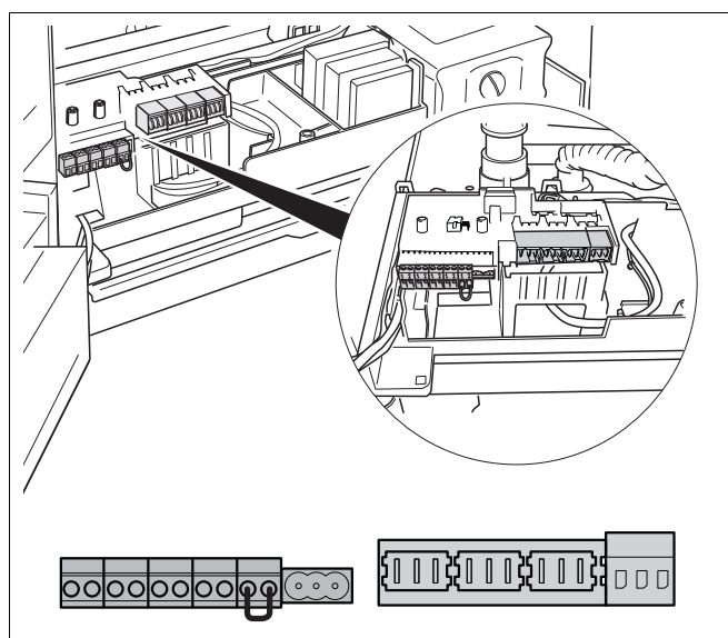
Рис. 24 Клеммная панель
