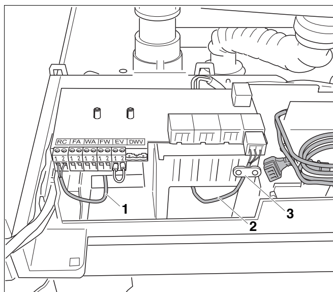
Рис. 25 Прокладка кабеля
