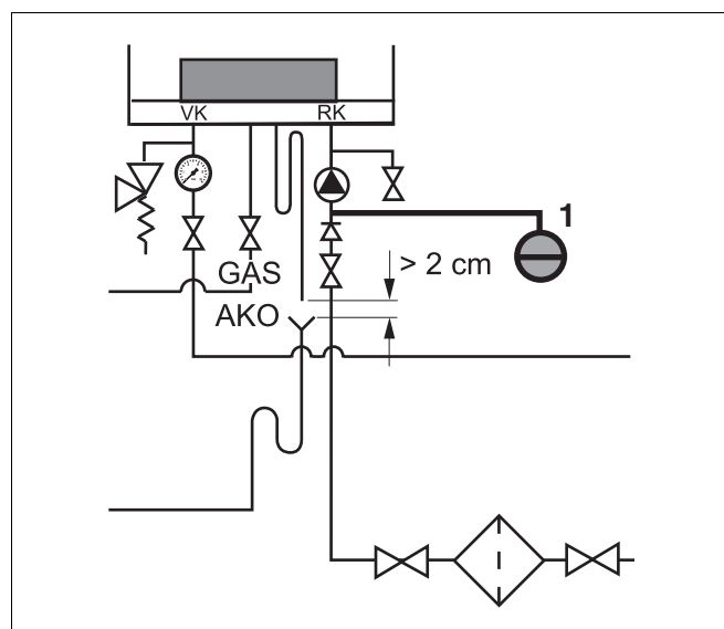
Рис. 21 Подключение расширительного бака в случае отдельного монтажа
